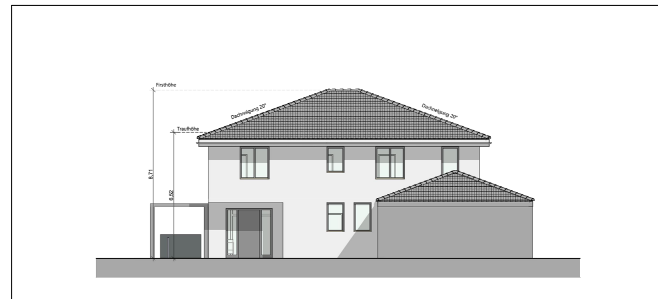
Ansicht Ost
