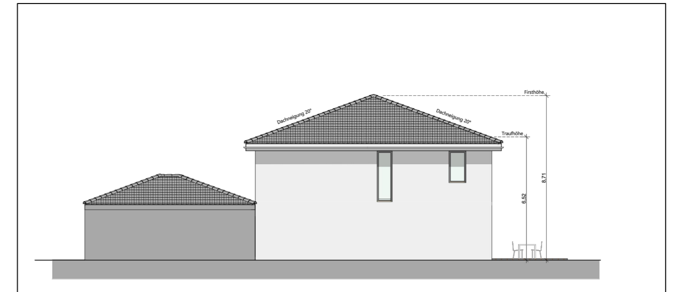
Ansicht Nord
