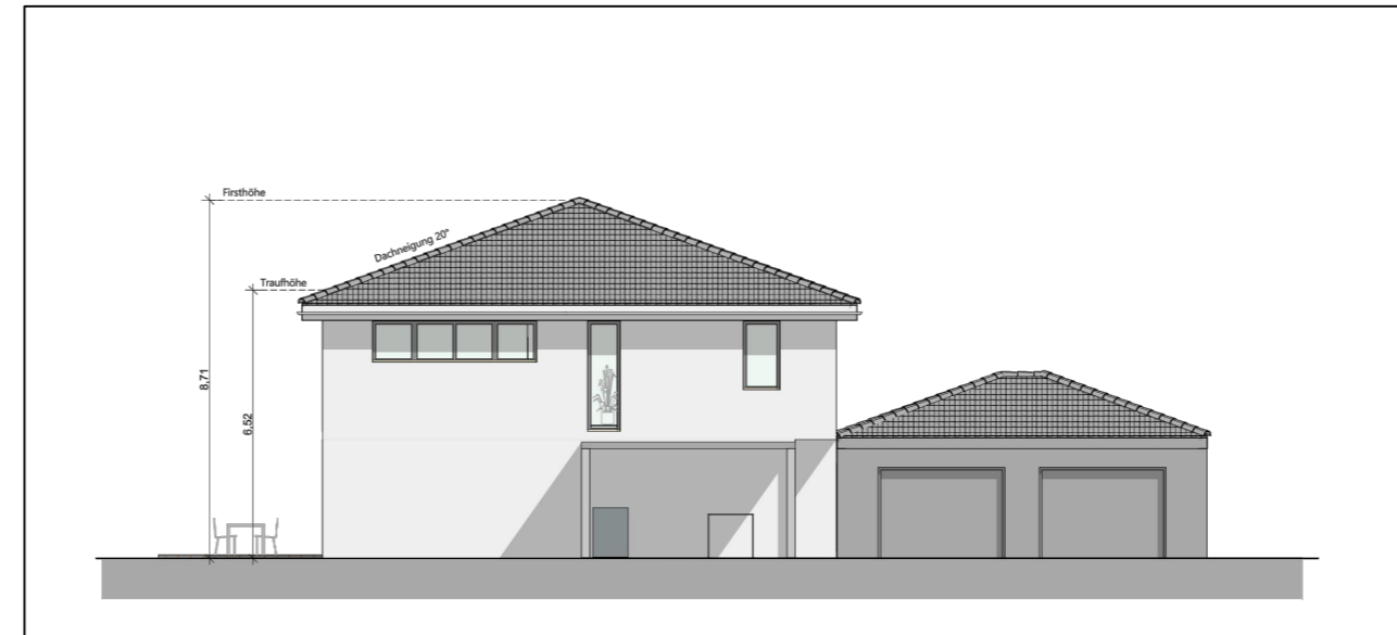
Ansicht Süd
